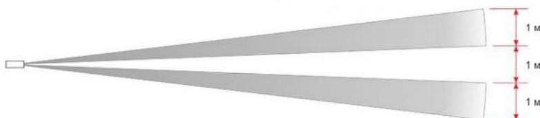
Зона обнаружения ИД2-50Ш
