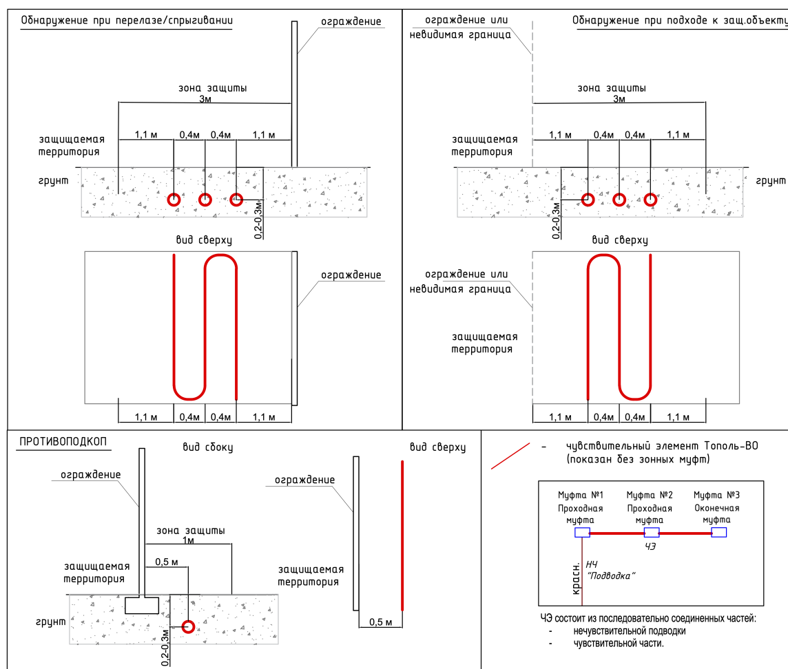
Варианты расположения чувствительного элемента (ЧЭ) "Тополь В0-КС" в грунте
