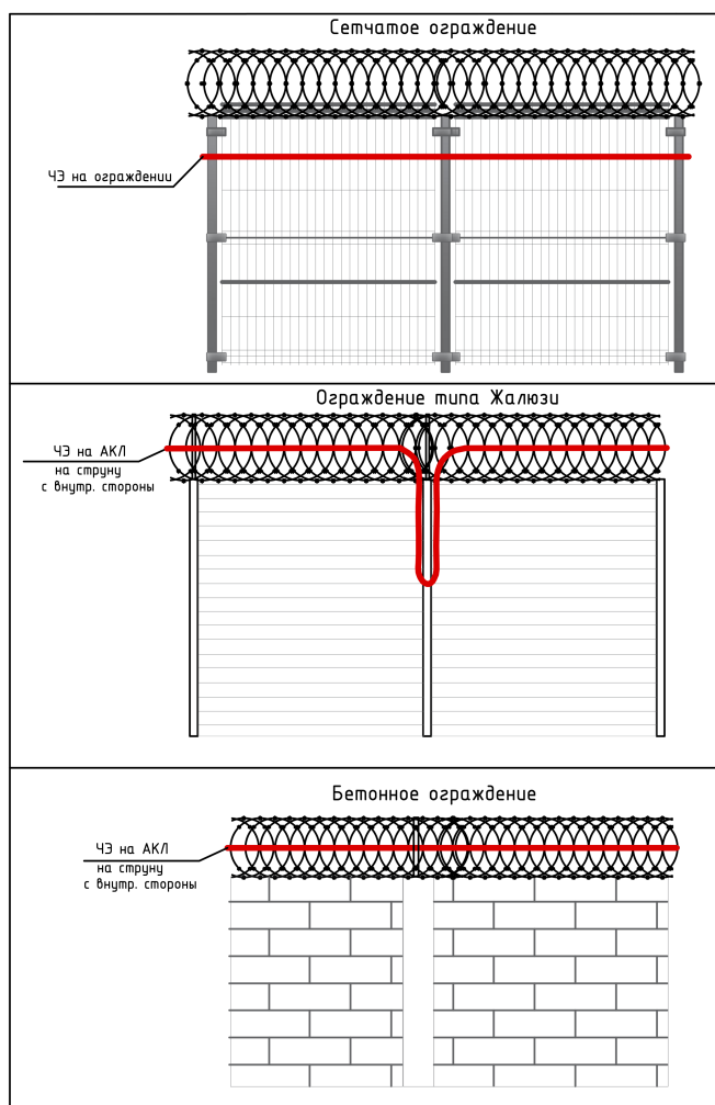
Одна зона на участок
