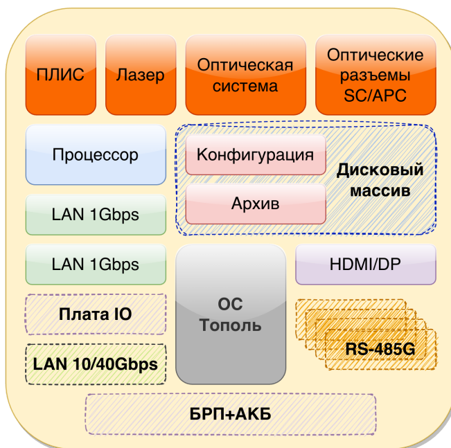
Блок обработки БОС-Ц-ВО
