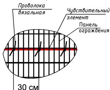
Схема крепления ЧЭ на панели ограждения
