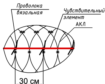
Схема крепления ЧЭ на АКЛ
