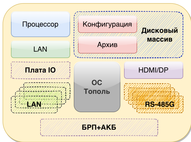
Блок обработки БОС-Ц
